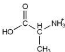
alaninium ion
