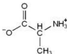
alanine (zwitterion notation)
