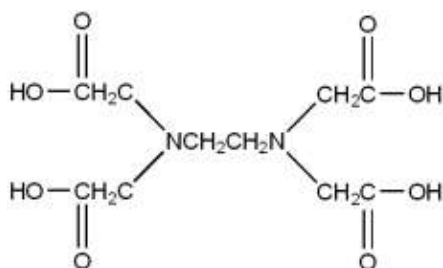
\text{H}_4\text{EDTA}
