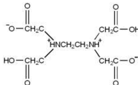
H_4EDTA (zwitterion)
