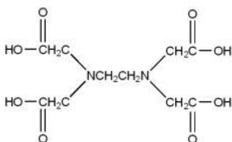
H_4EDTA (neutral)
